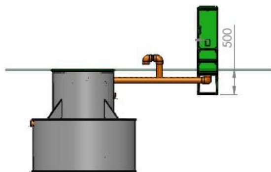
Billedet viser et 110 mm trækrør mellem den eksterne teknikkasse og renseanlægget. Placering som standard 5 meter fra renseanlægget.
